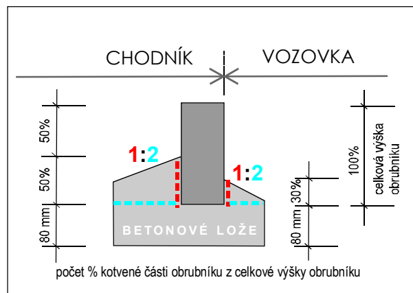
Základní schéma zabudování obrubníku
